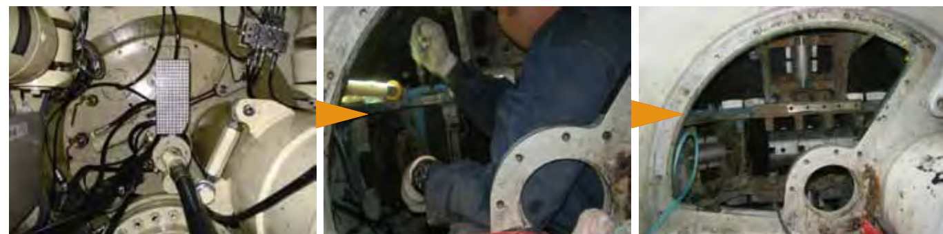
φ1,000mm 機内ビット交換状況
